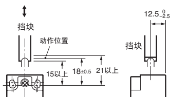
单侧悬臂滚珠摆杆型 (水平) (D4N-□□62)
