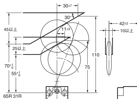
可调滚珠摆杆，锁定型 (金属摆杆，橡胶滚珠) (D4N-□□2H) (参考值)
