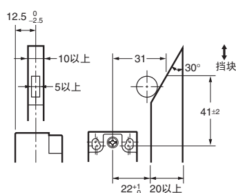
单侧悬臂滚珠摆杆型 (垂直) (参考值) (D4N-□□72)
