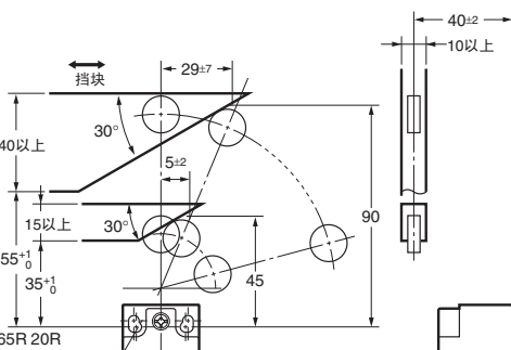
滚珠柱塞型 (D4N-□□32)
