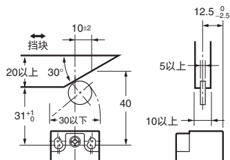
单侧悬臂滚珠摆杆型 (水平) (D4N-□□62)
