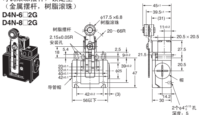
可调滚珠摆杆, 锁定型 (金属摆杆, 树脂滚珠)
