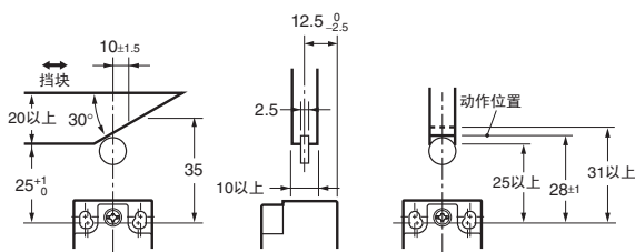
单侧悬臂滚珠摆杆型 (垂直) (参考值) (D4N-□□72)
