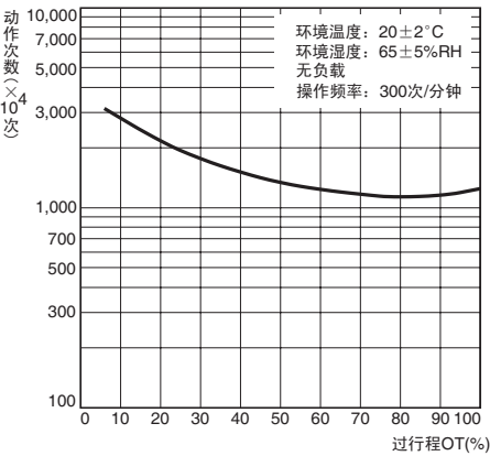
机械耐久性曲线(D2D-1000)
