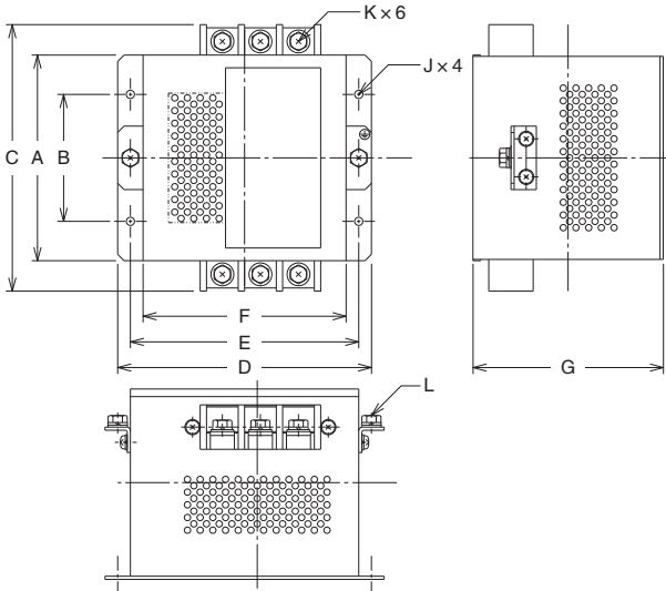
3G3AX-NFO03/3G3AX-NFO04/3G3AX-NFO05 3G3AX-NFO06
