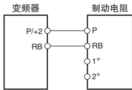
连接示例
