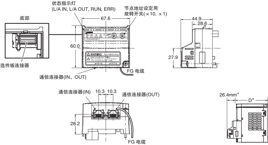
3G3AX–MX2–ECT
