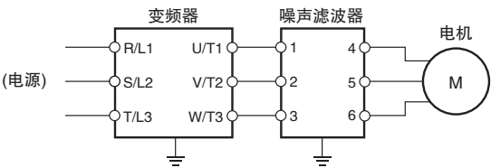
连接示例
