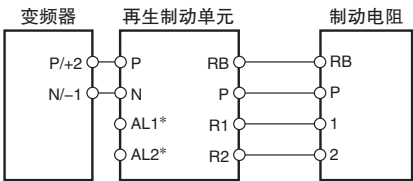
连接示例
