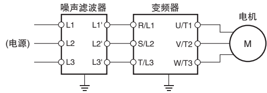
连接示例
