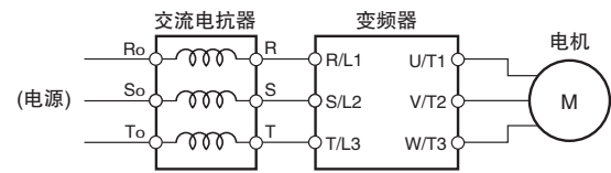
连接示例
