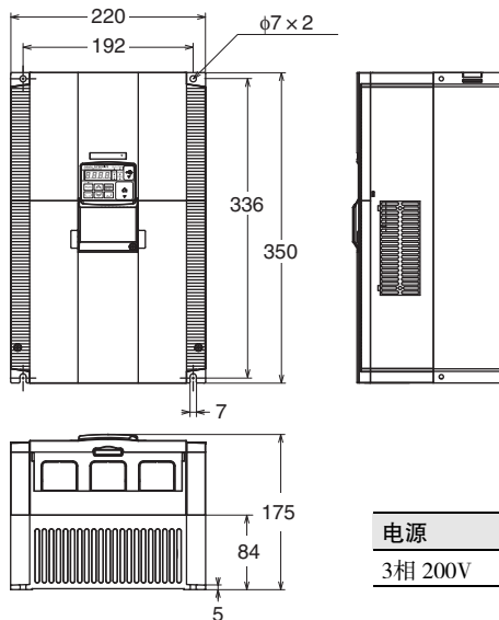
3G3MX2-A2150-ZV1
